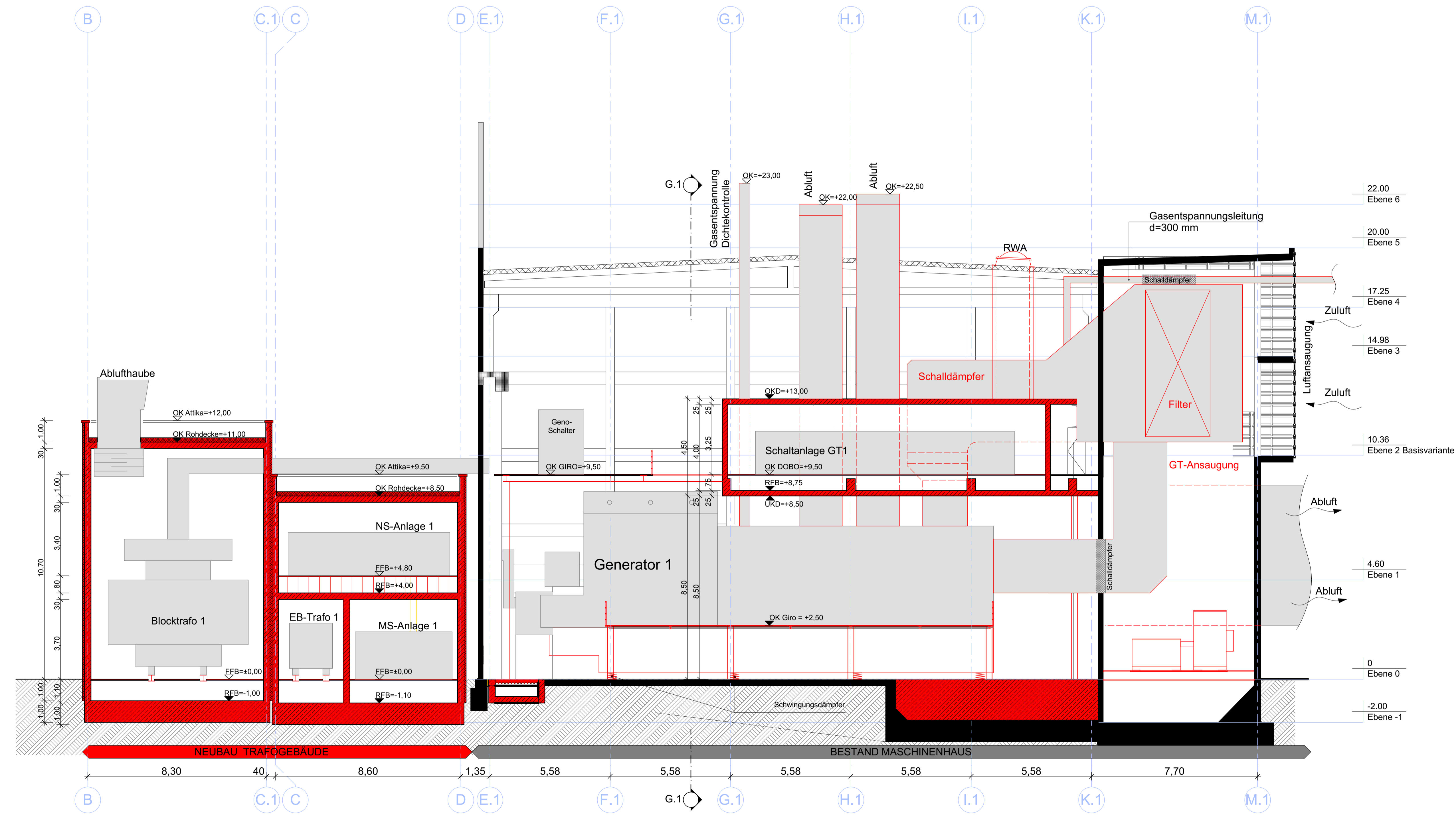
Schnitt Achse 6.1 - Maschinenhaus + Trafogebäude 1
